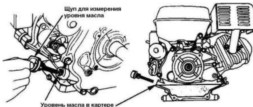
Рисунок 2 – Уровень масла в картере двигателя
