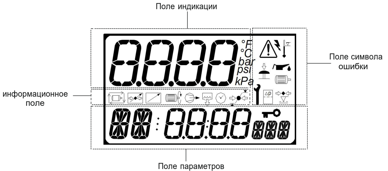
Рис. 1. Дисплей контроллера
