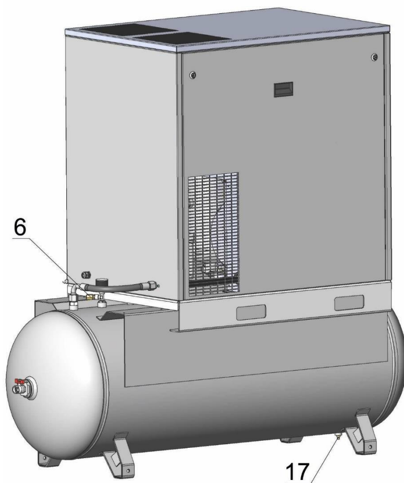
Рисунок 2 – Общий вид компрессорной установки BK20T-8(10,15)-500
